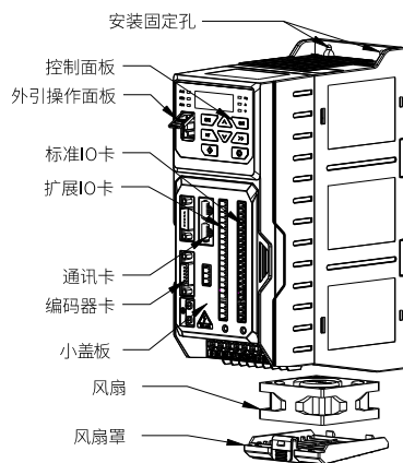
a) GK900-4T15LB 及以下
