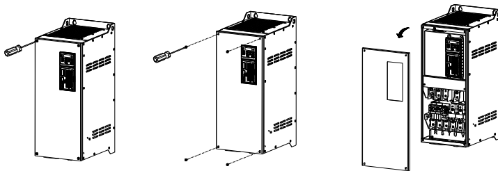
图 3-8 盖板的拆卸
