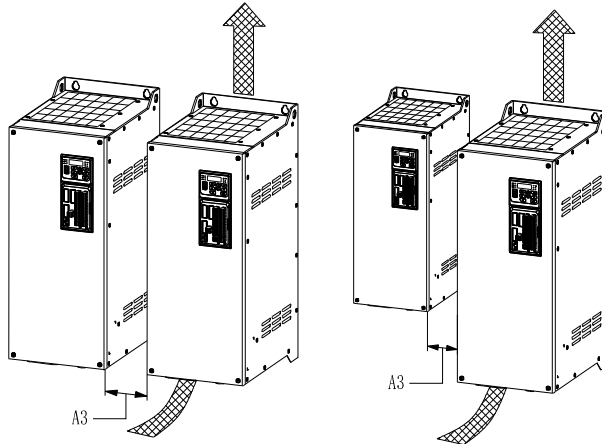
图 3-3 GK900-4T0.75LB~GK900-4T500L 安装方向和空间要求
