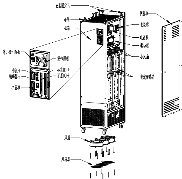
d) GK900-4T280L 及以上
