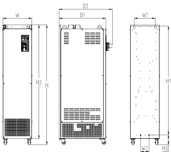
d) GK900-4T280L 及以上
