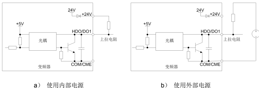
图 3-35 HDO 和 DO1 端子接上拉电阻输出时的接线方式
