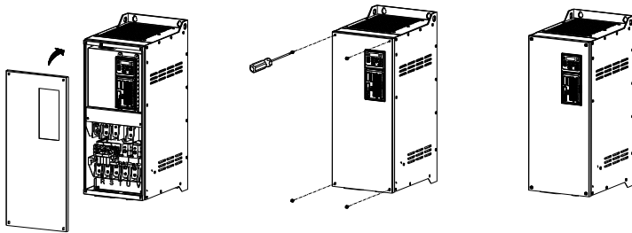
图 3-9 盖板的安装
