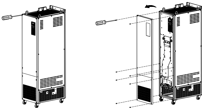
图 3-10 盖板的拆卸
