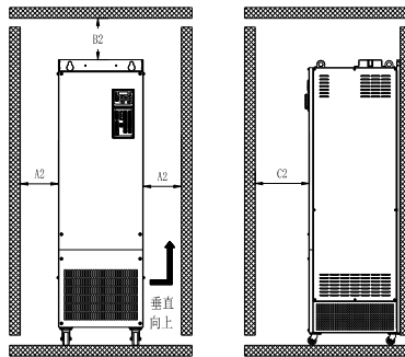
图 3-2 GK900-4T280L~GK900-4T500L 安装方向和空间要求
