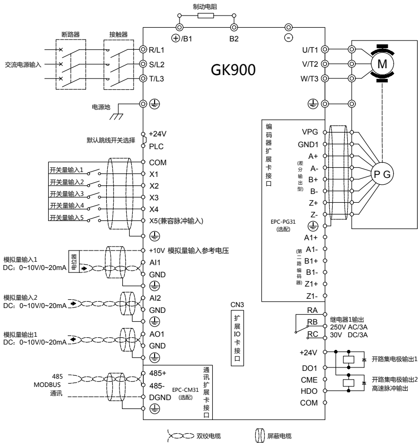
图 3-24 标准接线图
