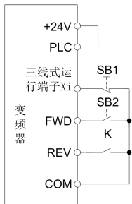
图 6-16 三线式模式 2
