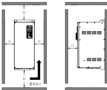
图 3-1 单台机器（GK900-4T0.75LB~GK900-4T250L）安装方向和空间
