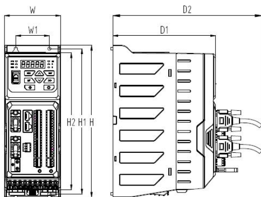
a) GK900-4T15LB 及以下
