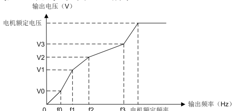
图 6-36 用户自定义多段 V/f 曲线
